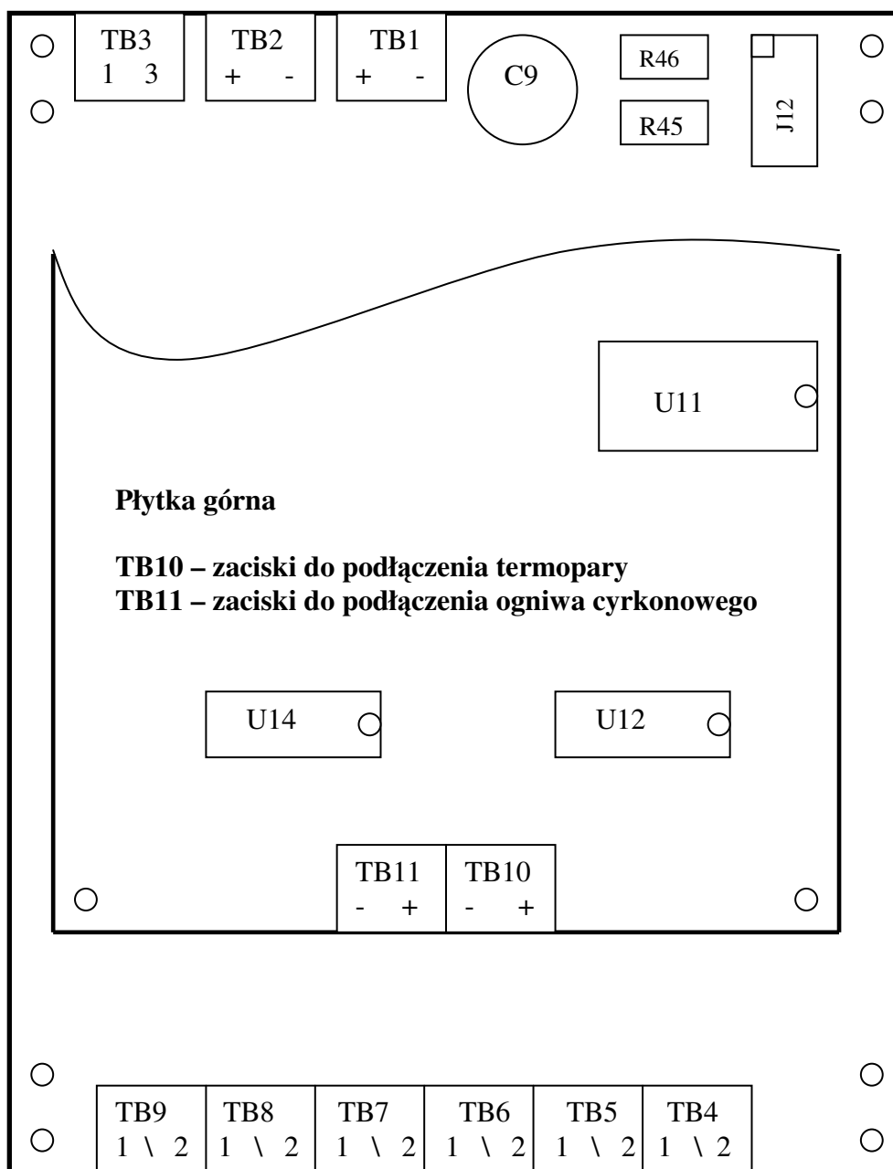
Rys. 4.1. Widok zacisków przyłączeniowych na płytkach drukowanych analizatora
